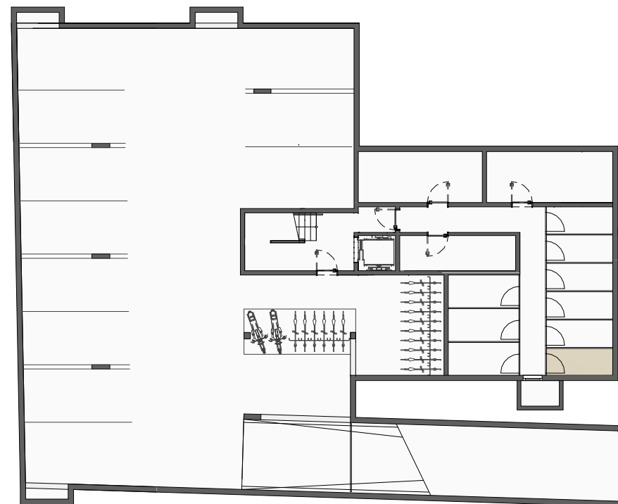
Übersicht Untergeschoss
