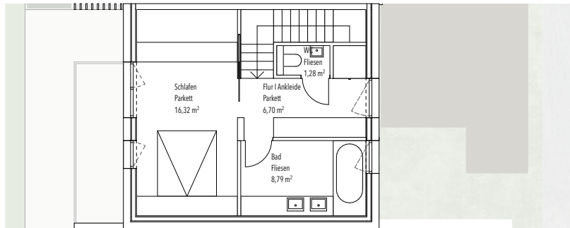
OBERGESCHOSS
