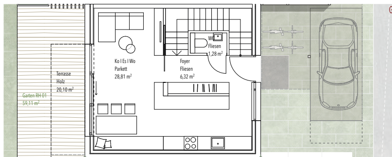
ERDGESCHOSS
