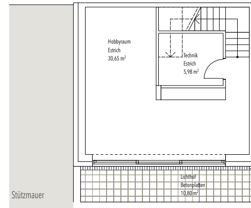
UNTERGESCHOSS
